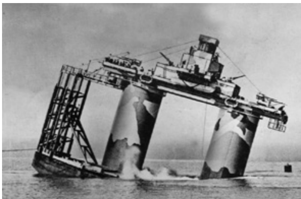
Roughs Tower s'assoit sur le fond de la mer en remplissant d'eau le ponton inférieur.
